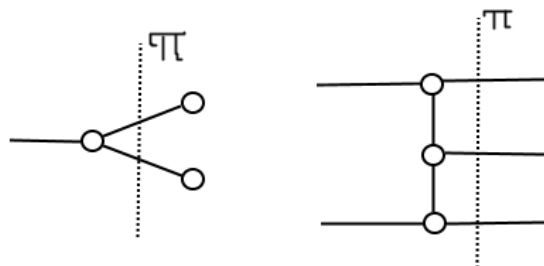
Obr. 2.2: Jednoduché príklady 1-pomocných množín typu 1. a 2.
