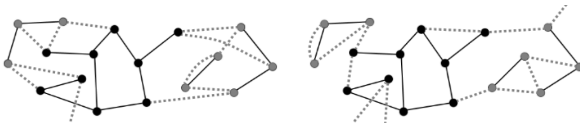
Obr. 2.1: Príklad tenkého a príklad hrubého čierneho komponentu pre \epsilon = 0,5
