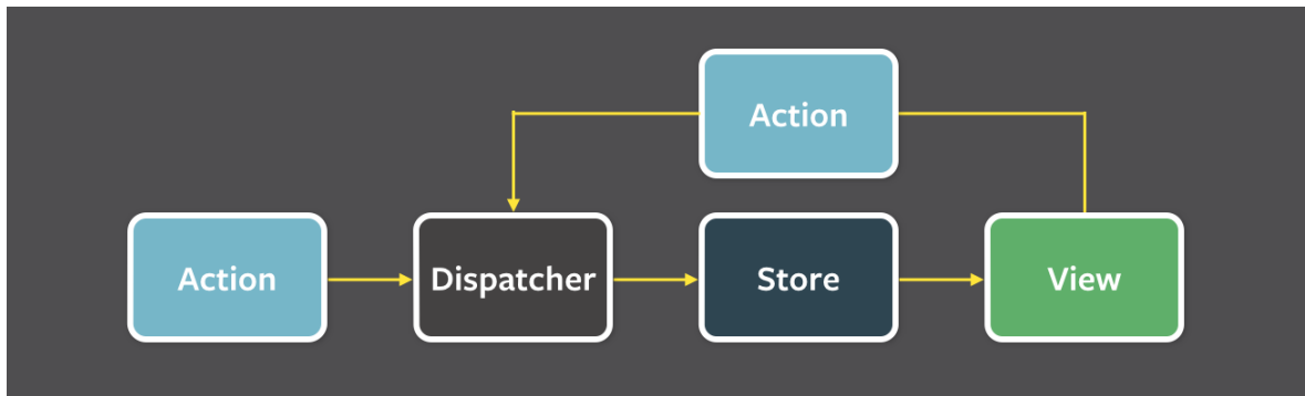
Obr. 3.1: Flux architektúra [13]
