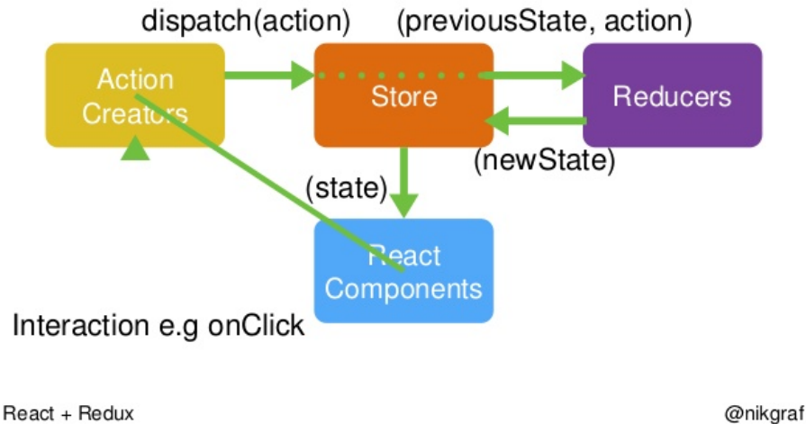
Obr. 3.2: Redux architektúra [21]
