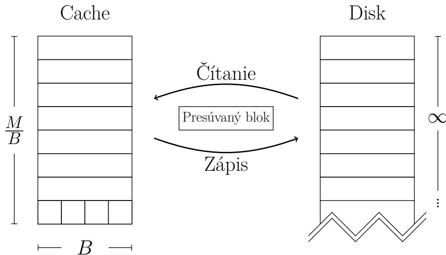
Obrázok 1.1: External-memory model
